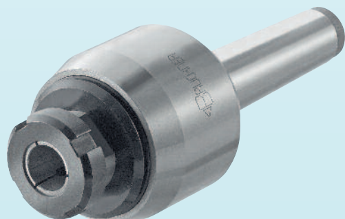
mit Spannzangenaufnahme
