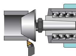
Form 258 für große Bohrungen
