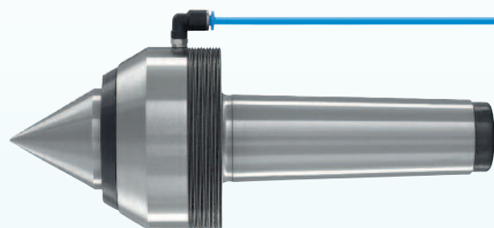
mit Sperrluftanschluss
