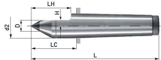
Form HE ähnlich DIN 806 HE
