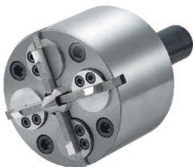
Stirnfutter HS mit hydraulischem Ausgleich
