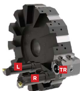
Внутреннее точение
